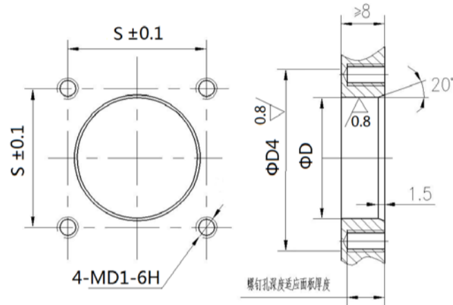
插座安装板开口尺寸
