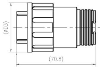
TKLC、TJLC 插头外形尺寸
