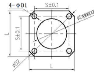
ZJBC、ZKBC 插座外形尺寸
