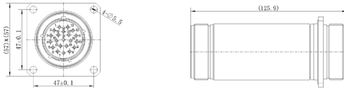
图 B.4 YS6-2321Z1DB 穿舱插座外形尺寸 (安装板开口尺寸见图 B.2)
