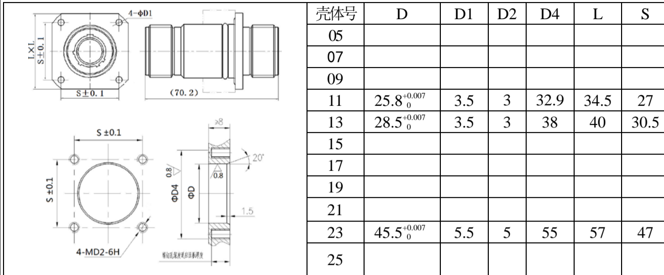
图 B.2 YS6 系列 ZCB、ZDB 穿舱插座外形尺寸
