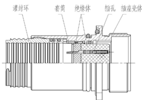
YS6系列灌封硫化插座
