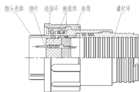
YS6系列灌封硫化插头
