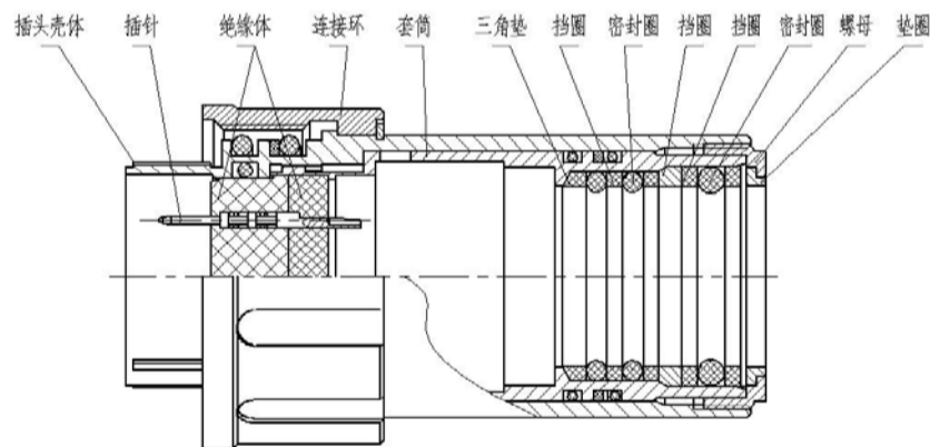
YS6系列挤压密封插头
