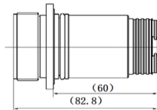
ZJBC、ZKBC 插座外形尺寸
