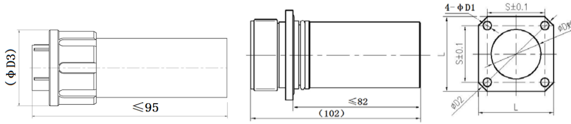
TKLA、TJLA 插头外形尺寸
