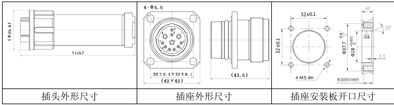
图 B.6 YS6 - 1711TJLA14/ZKB 外形尺寸 (单位为毫米)
