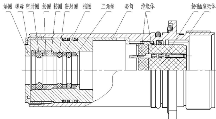
YS6系列挤压密封插座
