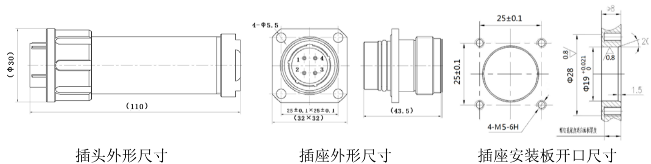
图 B.5 YS6-1104TJLA10/ZKB、YS6 II-1104TJLA10/ZKB 外形尺寸 (单位为毫米)
